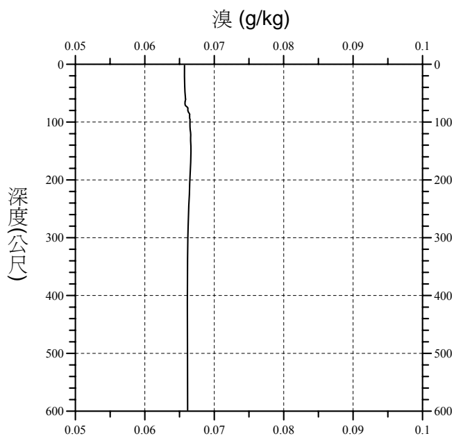
圖 1 台灣東岸台東知本深層海水溴離子濃度隨深度變化之實例（現場觀測日期、位置與海底深度：2006 年 10 月 12 日、121.0633°E；22.6437°N、650 m）。
