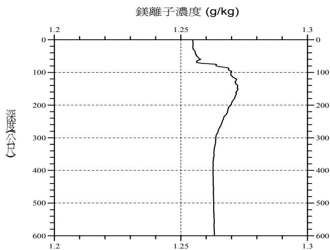
圖 1 台灣東岸台東知本深層海水鎂離子濃度隨深度變化之實例（現場觀測日期、位置與海底深度：2006 年 10 月 12 日、121.0633°E；22.6437°N、650 m）
