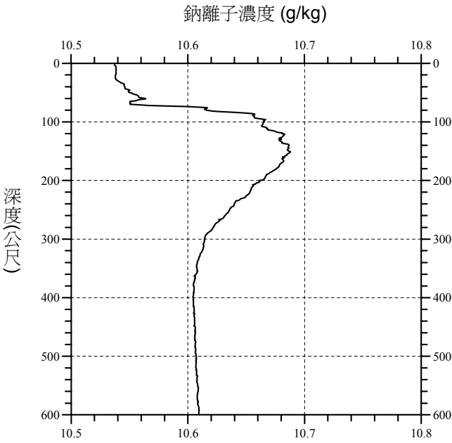
圖 1 台灣東岸台東知本深層海水鈉離子濃度隨深度變化之實例（現場觀測日期、位置與海底深度：2006 年 10 月 12 日、121.0633°E；22.6437°N、650 m）
