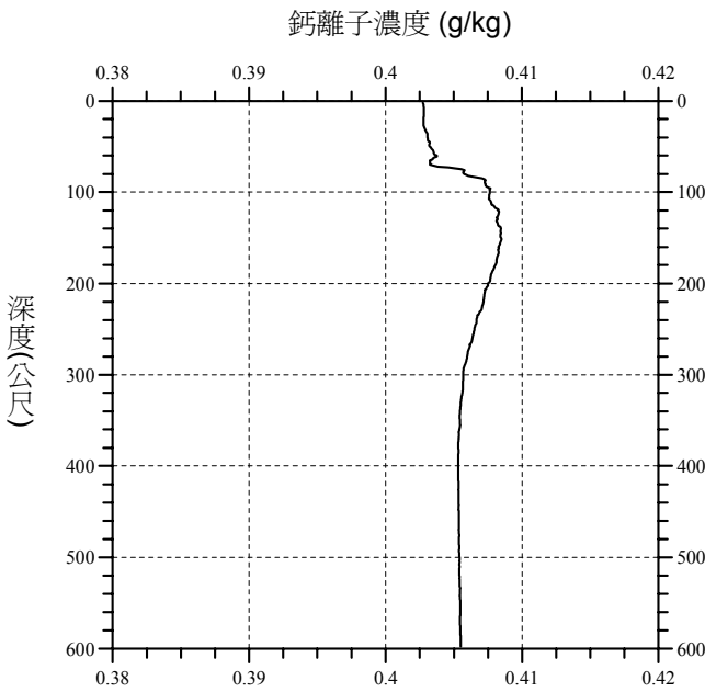
圖 1 台灣東岸台東知本深層海水鈣離子濃度隨深度變化之實例（現場觀測日期、位置與海底深度：2006 年 10 月 12 日、121.0633°E；22.6437°N、650 m）
