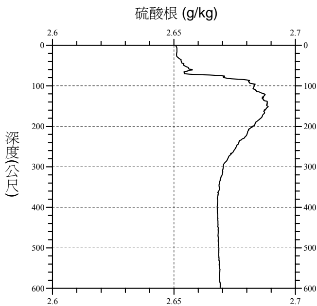
圖 1 台灣東岸台東知本深層海水硫酸根離子濃度隨深度變化之實例（現場觀測日期、位置與海底深度：2006 年 10 月 12 日、121.0633°E；22.6437°N、650 m）。
