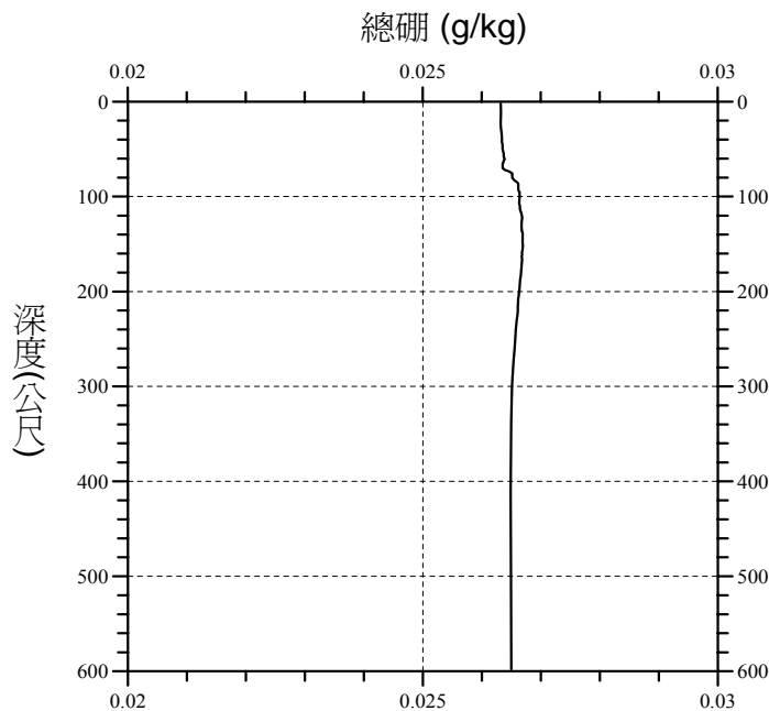
圖 1 台灣東岸台東知本深層海水總硼濃度隨深度變化之實例（現場觀測日期、位置與海底深度：2006 年 10 月 12 日、121.0633°E；22.6437°N、650 m）。
